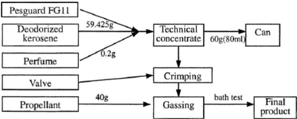
Рисунок 6-11 Процесс заполнения 0,3%-ного аэрозоля-инсектицида на масляной основе Pesguard
