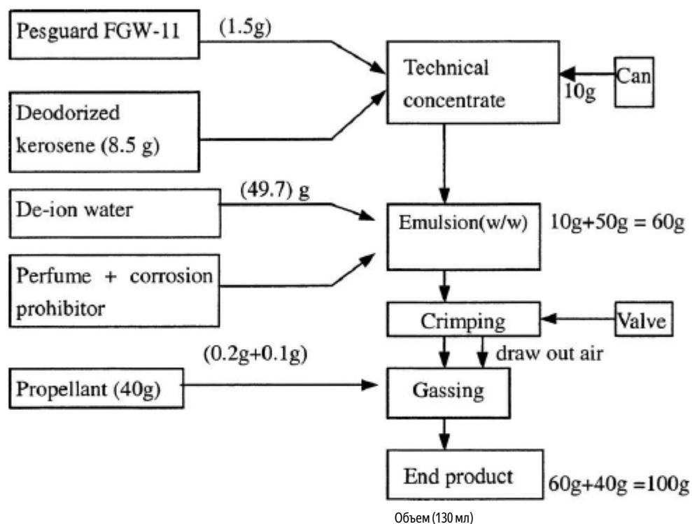
Рисунок 6-12 Процесс получения аэрозоля на водной основе FGW-11 (T-t-V)
