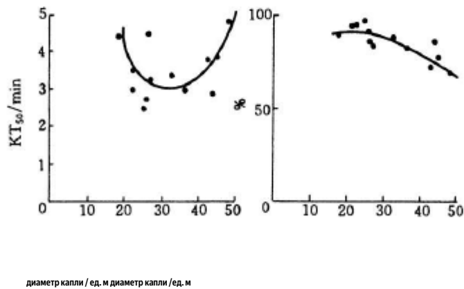
Рисунок 6-29 Взаимосвязь между диаметром капли и эффективностью для насекомых
