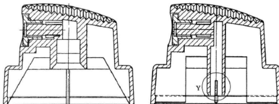
Рисунок 6-9 Привод для использования Рисунок 6-10 Привод для использования с охватывающим клапаном с охватывающим клапаном
