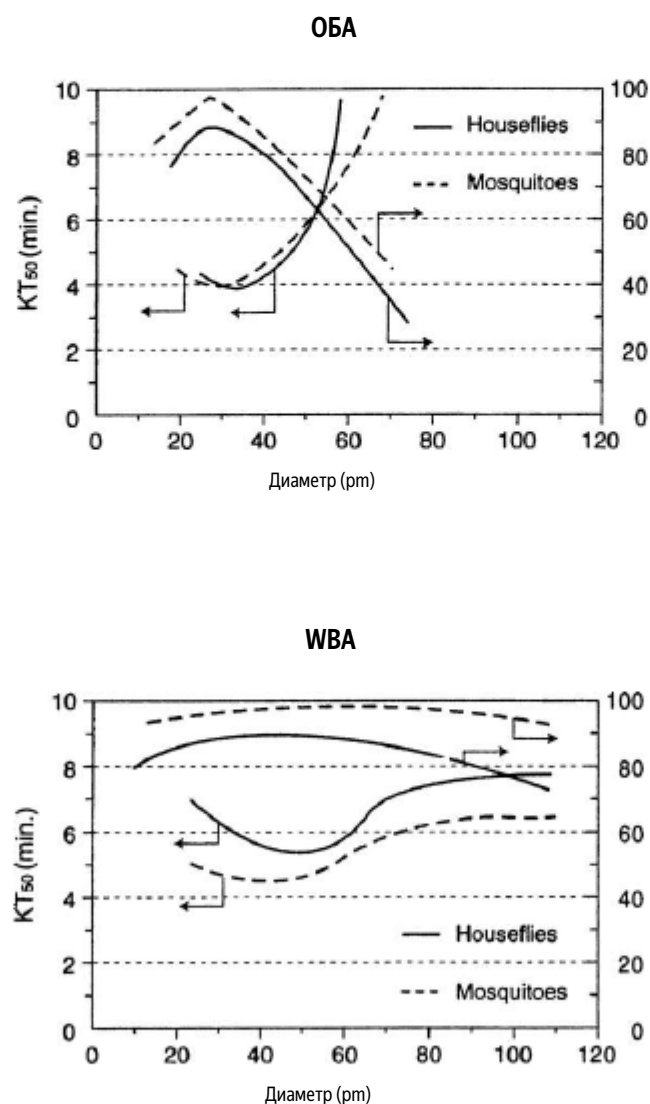
Рисунок 6-26 Взаимосвязь между размером капель и эффективностью аэрозолей WBA и ОВА в борьбе с мухами и комарами
