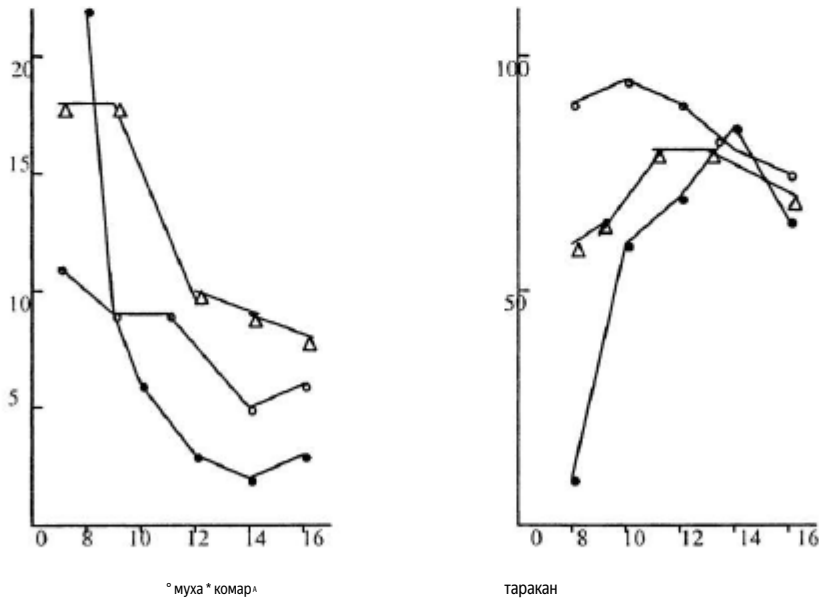
Рисунок 6-4 Диапазон чисел атомов углерода растворителей в зависимости от сбивающего действия и летального эффекта и аэрозоля от комаров до 5,8 м³ примечание к камере- 1. Для борьбы с мухами 2. Для борьбы с тараканами распылите непосредственно в стеклянный цилиндр (20 см в диаметре, 60 см в высоту).
