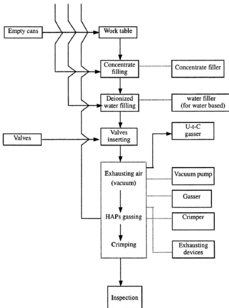
Рисунок 6-15 Заполнение методом U-t-C
