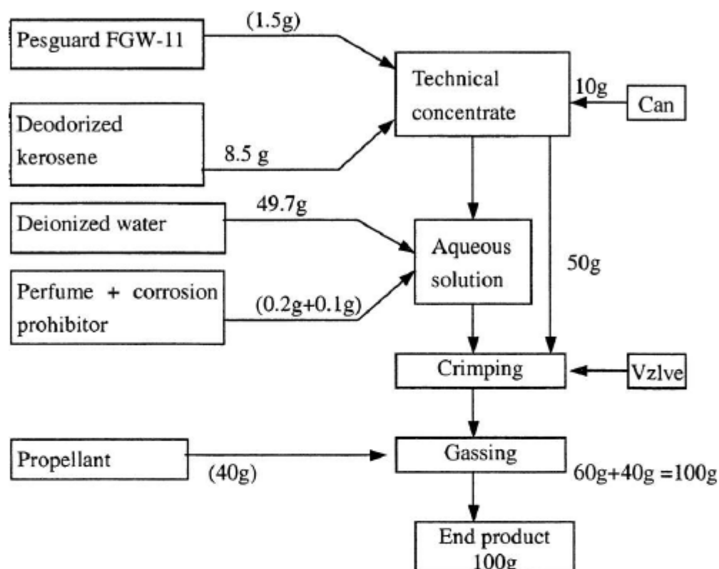
Рисунок 6-13 - Процесс получения аэрозоля на водной основе FGW 11
