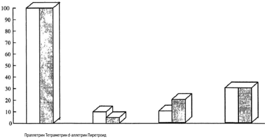
Праллетрин Тетраметрин d-аллетрин Пиретроид
