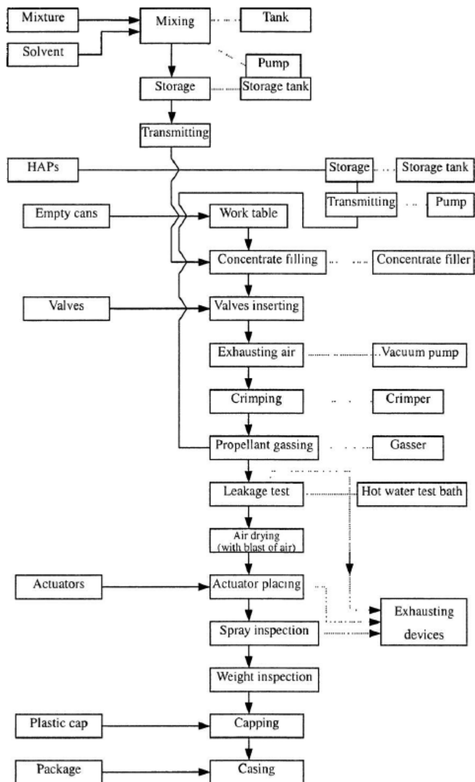
Рисунок 6-16 Процесс получения инсектицидных аэрозолей на масляной основе (Т-т-В)
