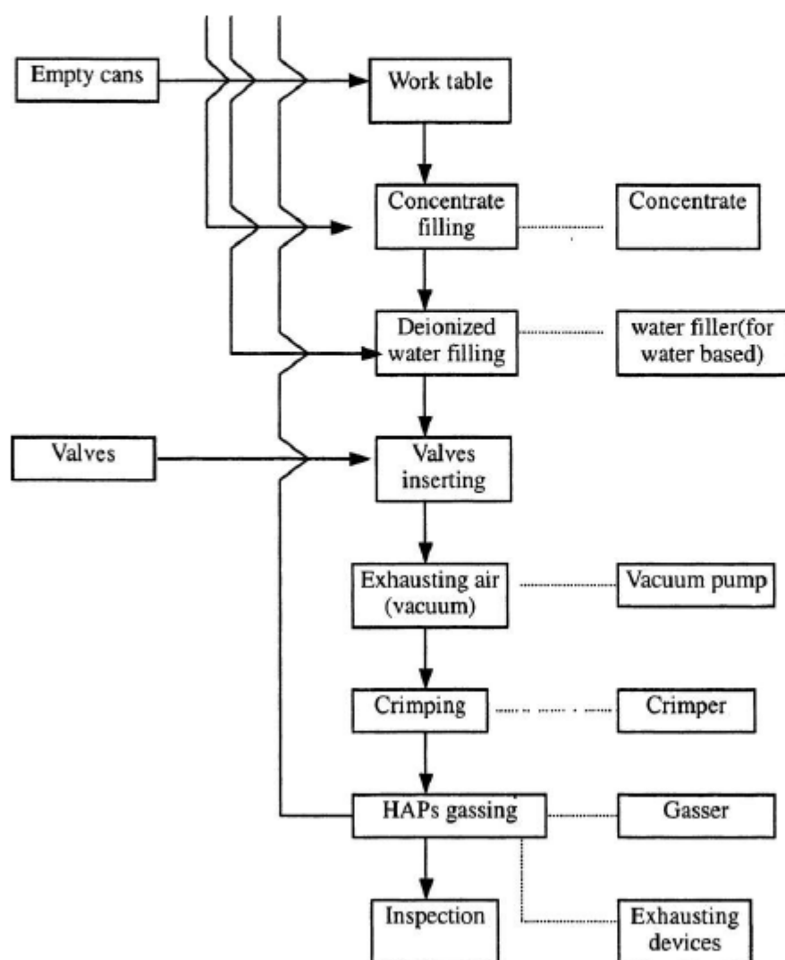
Рисунок 6-14 Заполнение методом T-t-V.
